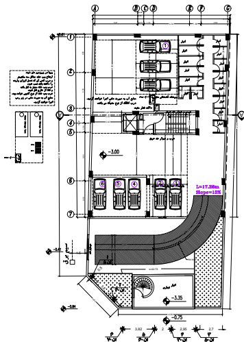
پلان زیر زمین -1 1:100
