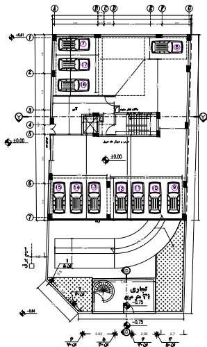
پلان طبقه همکف 1:100
