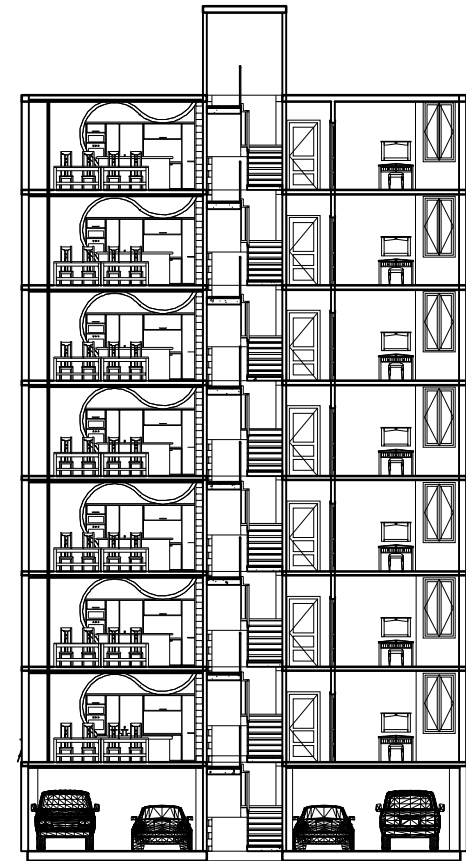
برش A-A
